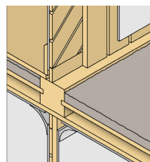
Bræddeskillevæg
