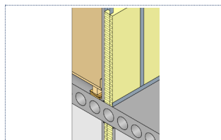
Let væg
