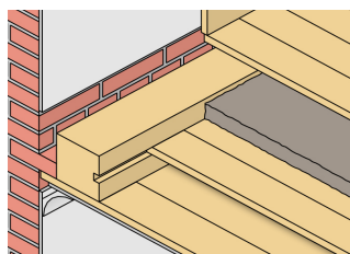
Træetageadskillelse
