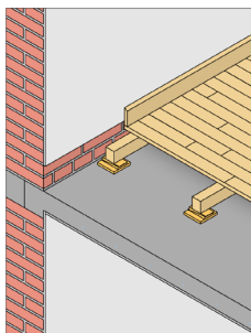
Støbt beton
