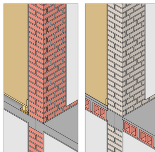
Murede vægge
