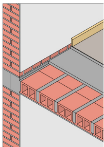
Tegldæk
